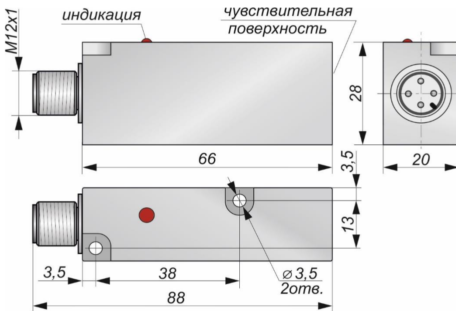
Габаритный чертеж
