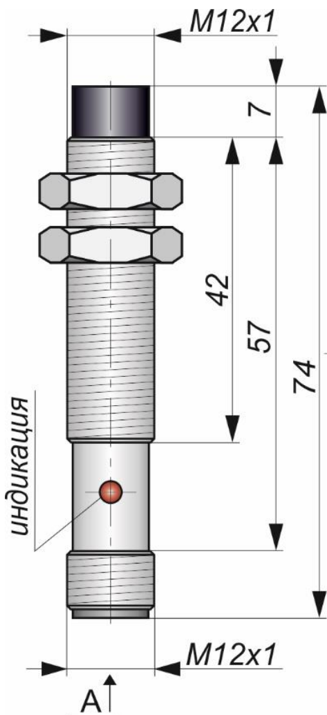
Габаритный чертеж
