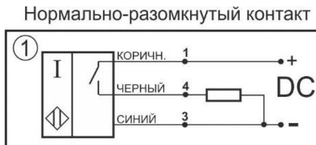
Схема соединения
