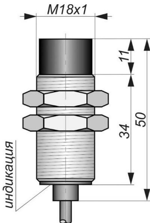
Габаритный чертеж
