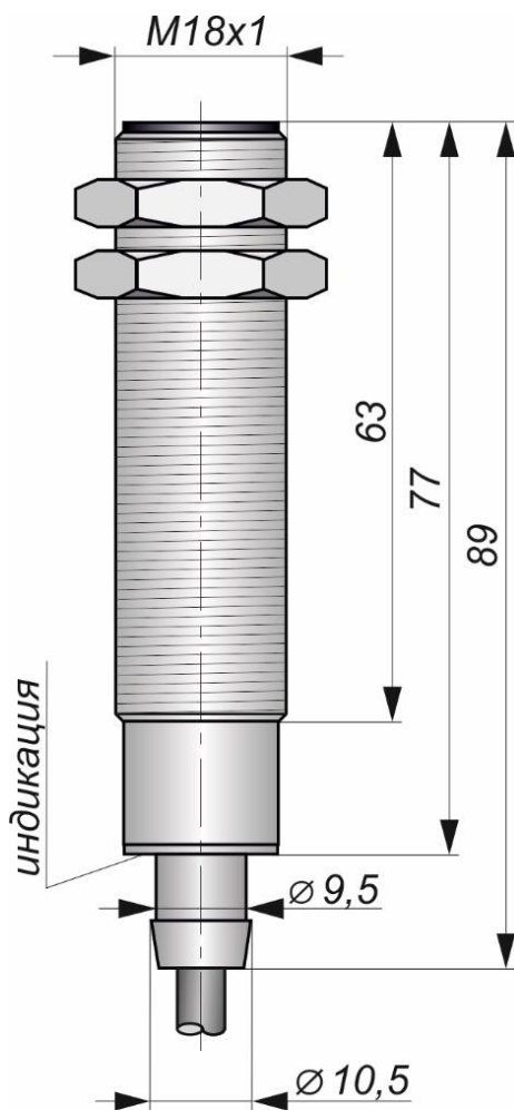
Габаритный чертеж
