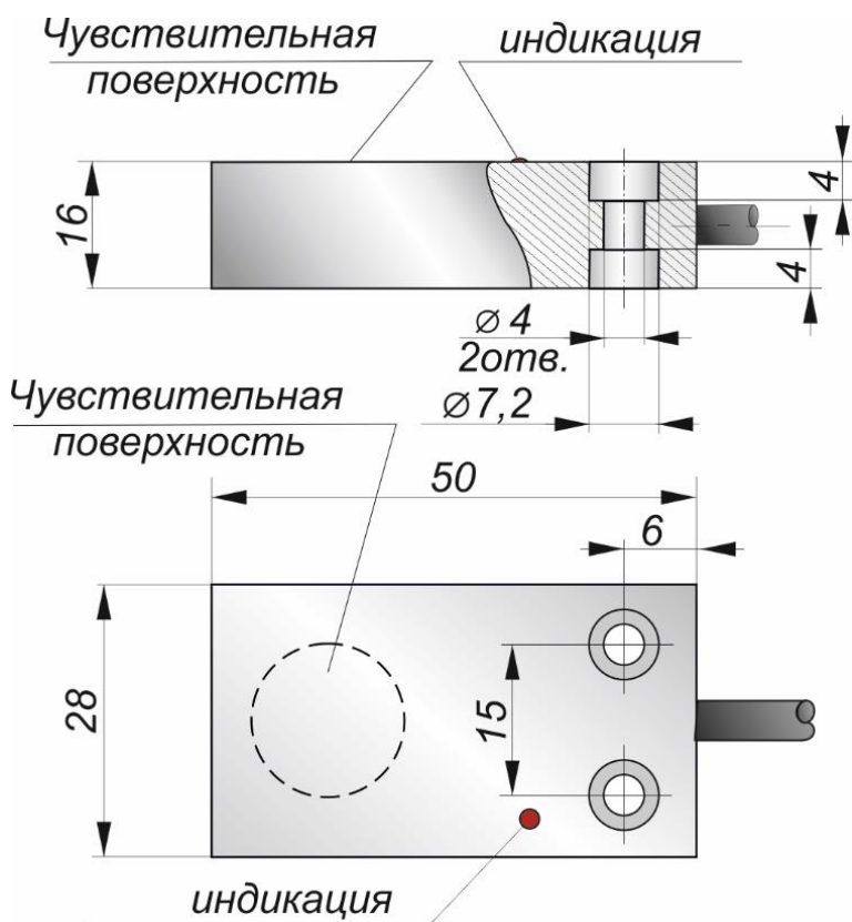
Габаритный чертеж
