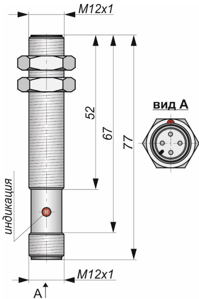
Габаритный чертеж
